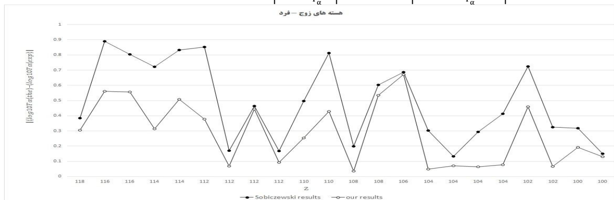
شکل ۲: نمودار \left| \log_{10}\left(\frac{T_{\alpha}^{Sobiczewski}}{T_{\alpha}^{exp}}\right) \right| (دایره های توپر) و \left| \log_{10}\left(\frac{T_{\alpha}^{My}}{T_{\alpha}^{exp}}\right) \right| (دایره های توخالی) برای هسته های زوج-فرد (Z(even)-N(odd))
