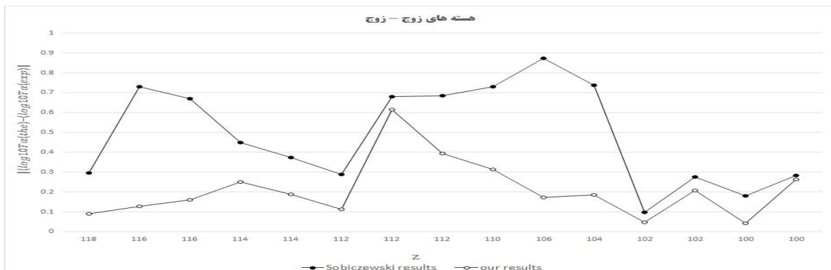
شکل ۱: نمودار \left| \log_{10}\left(\frac{T_{\alpha}^{Sobiczewski}}{T_{\alpha}^{exp}}\right) \right| (دایره های توپر) و \left| \log_{10}\left(\frac{T_{\alpha}^{My}}{T_{\alpha}^{exp}}\right) \right| (دایره های توخالی) برای هسته های زوج-زوج (Z(even)-N(even))
