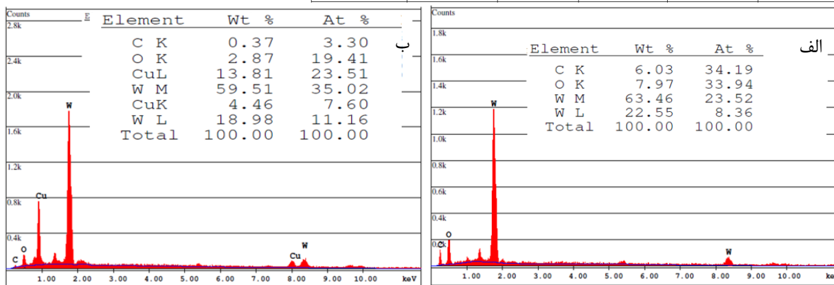
شکل ۶: نتایج آنالیز EDX از نمونه‌ی تنگستن (الف) قبل از پرتو دهی، (ب) بعد از پرتو دهی
