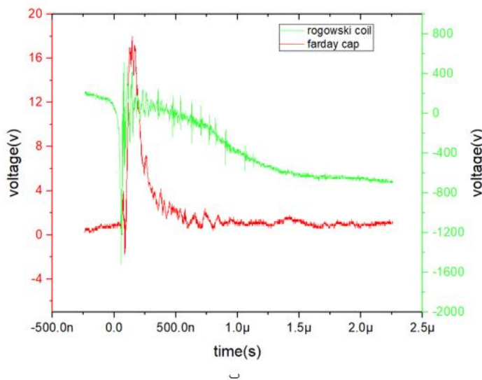
شکل ۲: الف) فنجان فارادی درون نگهدارنده ب) سیگنال قرمز، سیگنال حاصل از فنجان فارادی و سیگنال سبز سیگنال ناشی از پیچ‌های روگوفسکی می‌باشد.
