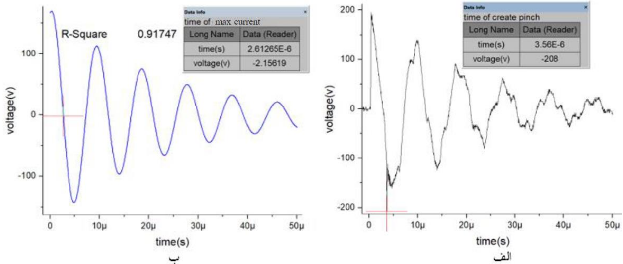
شکل ۱: الف) سیگنال تخلیه جریان که توسط پیچ‌های روگوفسکی روی نوسان‌نما ثبت شده، ب) نمودار برازش شده به سیگنال تخلیه‌ی جریان
