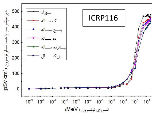
شکل ۴. مقادیر دوز موثر بر حسب انرژی نوترون برای ۶ گروه سنی در هندسه پرتوگیری پشت و با W_R های منتشر شده در ICRP های مختلف
