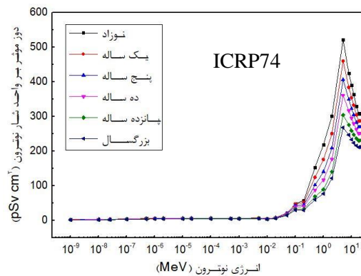
شکل ۵. مقادیر دوز موثر بر حسب انرژی نوترون برای ۶ گروه سنی در هندسه پرتوگیری سمت راست و با W_R های منتشر شده در ICRP های مختلف
