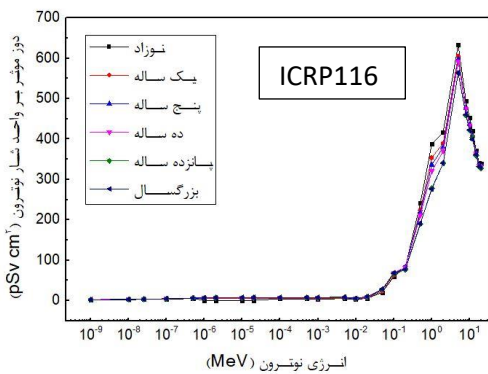
شکل ۲. مقادیر دوز موثر بر حسب انرژی نوترون برای ۶ گروه سنی در هندسه پرتوگیری رو به رو و با W_R های منتشر شده در ICRPهای مختلف
