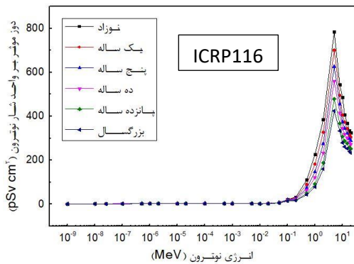
شکل ۳. مقادیر دوز موثر بر حسب انرژی نوترون برای ۶ گروه سنی در هندسه پرتوگیری سمت چپ و با W_R های منتشر شده در ICRPهای مختلف
